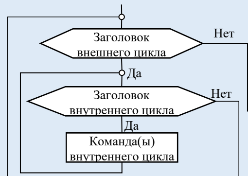
Пример 13.4. Блок-схема вложенных циклов.
